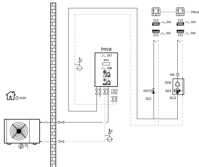
Ilustracja 5.2. Schemat instalacji INTRA HEX z dwustrefowym systemem ogrzewania/chłodzenia
