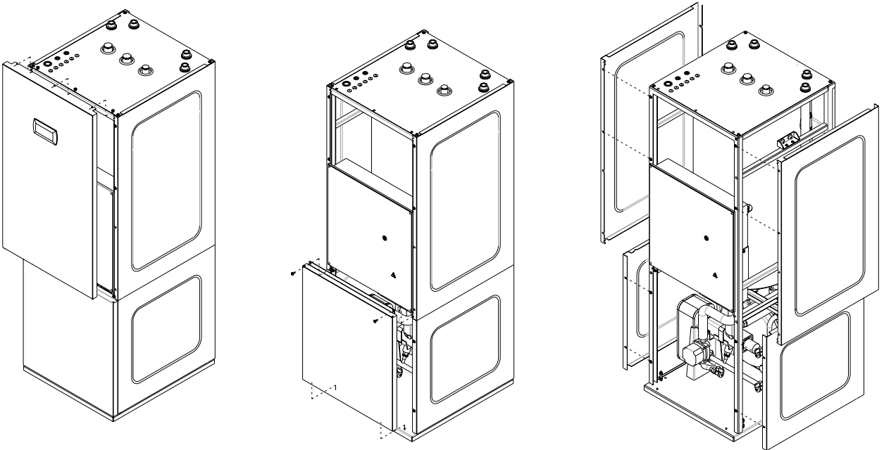
Ilustracja 4.3. Zdejmowanie osłony modułu wewnętrznego Intra BOOST.
