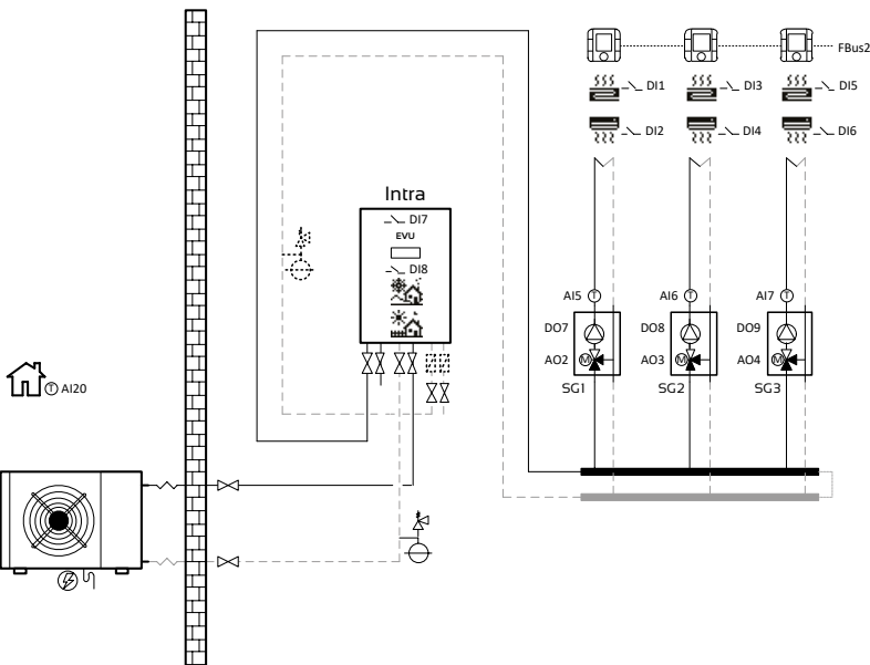
Ilustracja 5.3. Schemat instalacji INTRA HEX z trzema strefami ogrzewania/chłodzenia
