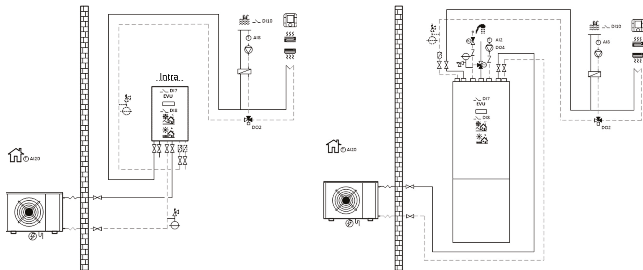
Ilustracja 5.7. Schemat połączeń obiegu ogrzewania wody w basenie z Intra HEX i Intra BOOST
