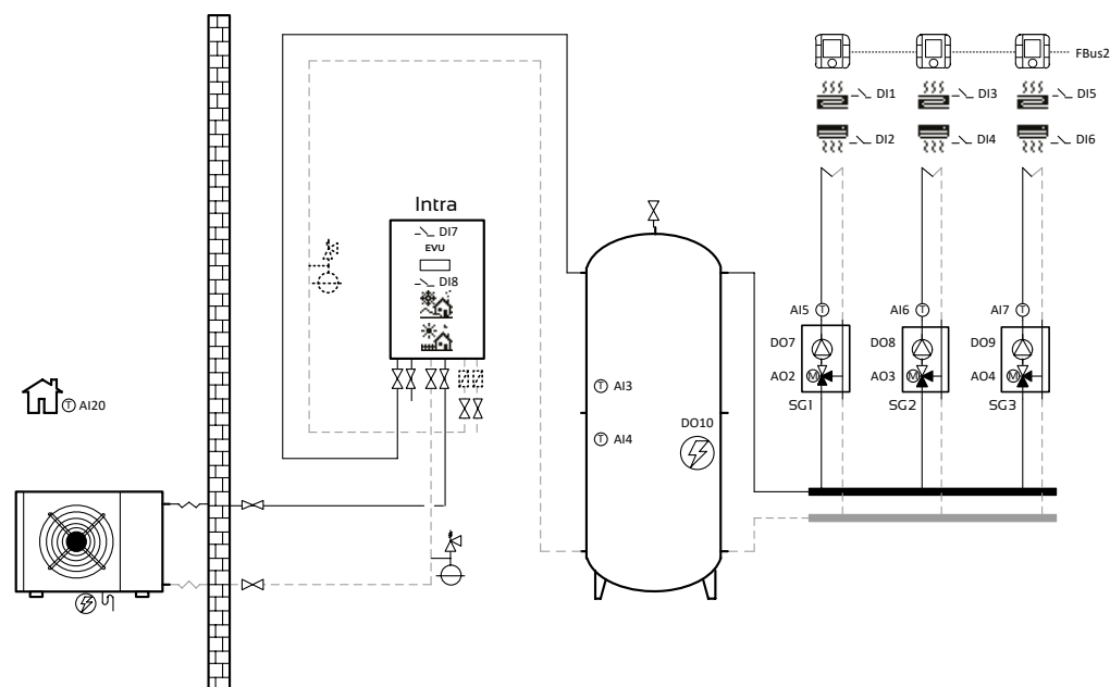
Ilustracja 5.5. Schemat połączeń poprzez jeden zasobnik buforowy
