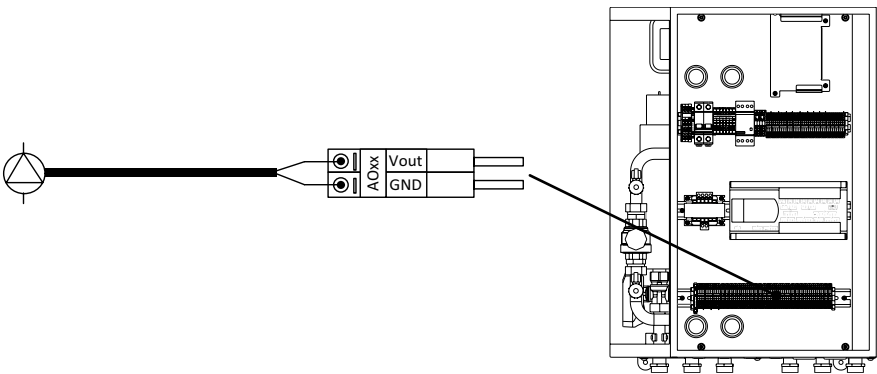
Ilustracja 7.6. Przykład podłączenia sygnału sterującego PWM.
