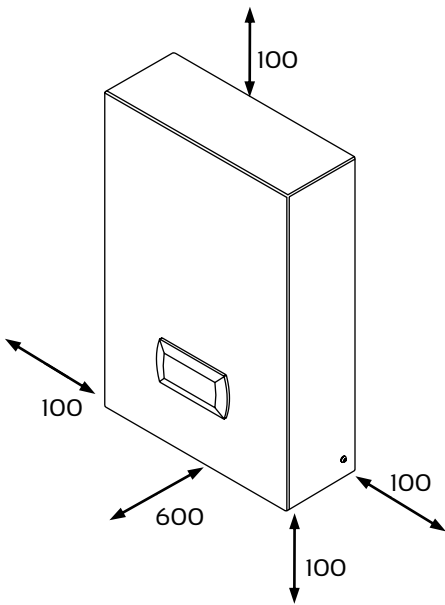
Ilustracja 2.4. Zalecane minimalne obszary serwisowe wokół modułu wewnętrznego Intra CONTROL (w mm).
