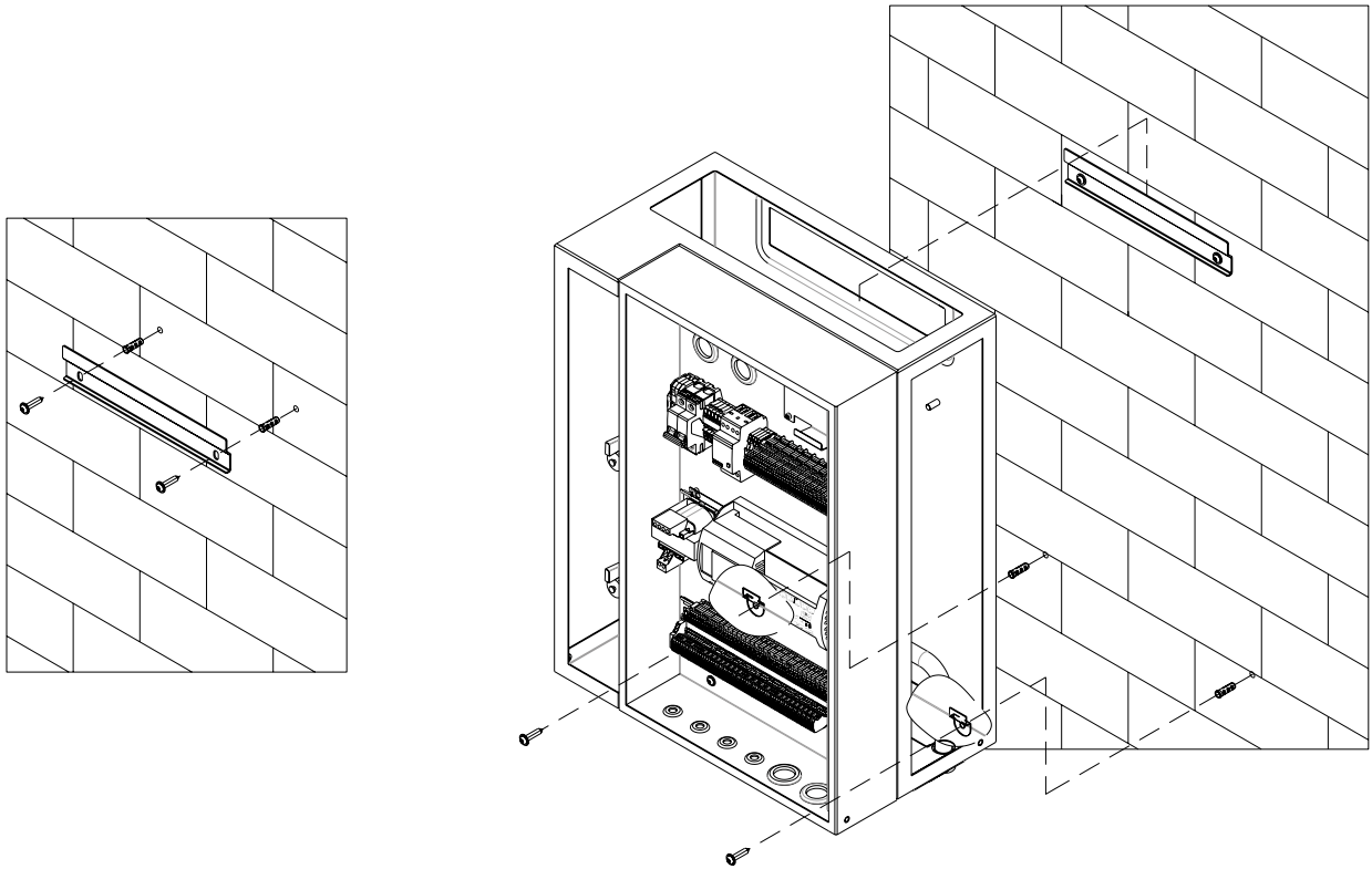
Ilustracja 3.4. Zakładanie modułów wewnętrznych Intra HEX.
