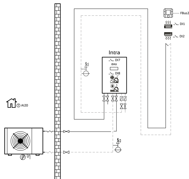
Ilustracja 5.1. Schemat instalacji INTRA HEX z jednostrefowym systemem ogrzewania/chłodzenia
