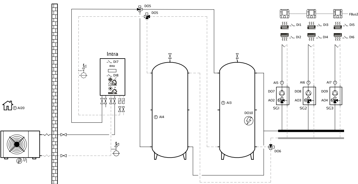
Ilustracja 5.4. Schemat instalacji z wykorzystaniem dwóch zbiorników buforowych
