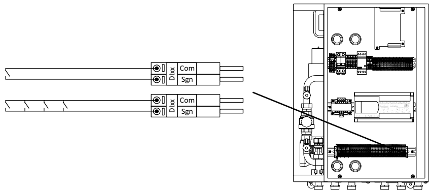
Ilustracja 7.11. Przykład podłączenia jednego termostatu i kilku równolegle.
