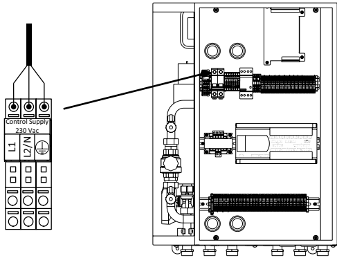
Ilustracja 7.9. Schemat połączeń obwodu zasilania elektrycznego modułu wewnętrznego.
