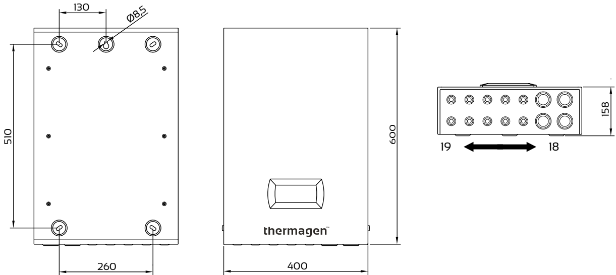
Ilustracja 2.1. Ogólne wymiary modułu wewnętrznego Intra CONTROL (w mm).
