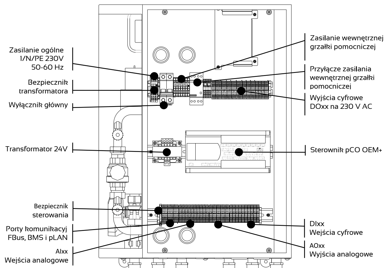
Ilustracja 7.1. Rozmieszczenie elementów tablicy elektrycznej (moduły wewnętrzne Intra CONTROL i Intra HEX/BOOST).
