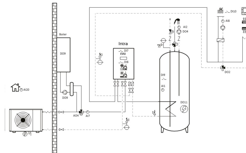
Ilustracja 5.8. Schemat połączenia kotła z modułem Intra HEX.
