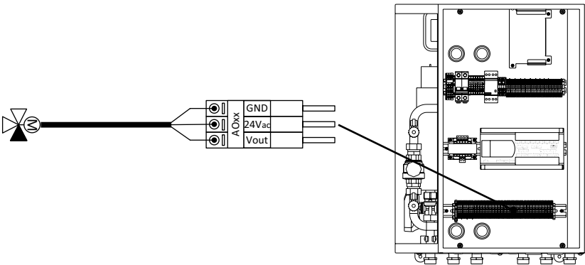
Ilustracja 7.7. Przykład podłączenia sygnału sterującego 0-10Vdc.
