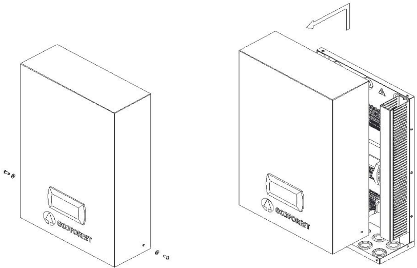
Ilustracja 2.2. Zdejmowanie przedniej osłony modułu wewnętrznego Intra CONTROL.
