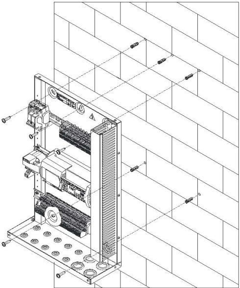
Ilustracja 2.3. Umieszczenie modułu wewnętrznego Intra CONTROL.
