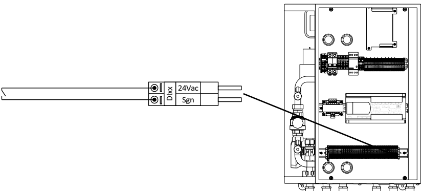
Ilustracja 7.5. Przykład podłączenia wejść cyfrowych z napięciem 24V AC.
