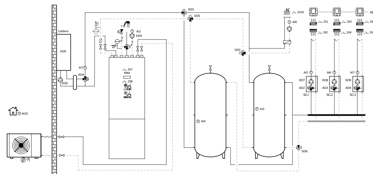
Ilustracja 7.2. Ogólny schemat połączeń elektrycznych modułu wewnętrznego
