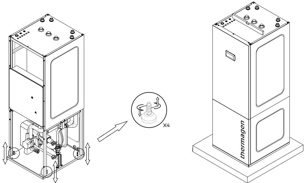
Ilustracja 4.4. Ustawianie i poziomowanie modułów wewnętrznych Intra BOOST.
