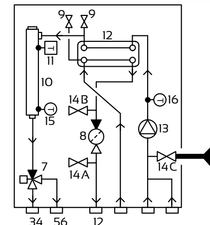
Ilustracja 6.2. Napełnianie obwodu pomocniczego z modułem wewnętrznym Intra HEX
