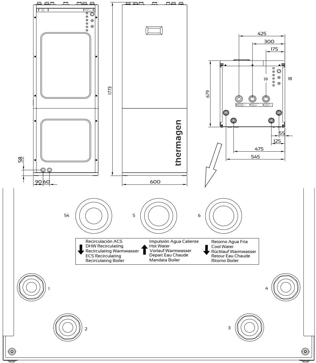
Ilustracja 4.1. Ogólne wymiary i połączenia hydrauliczne modułów wewnętrznych Intra BOOST (w mm).
