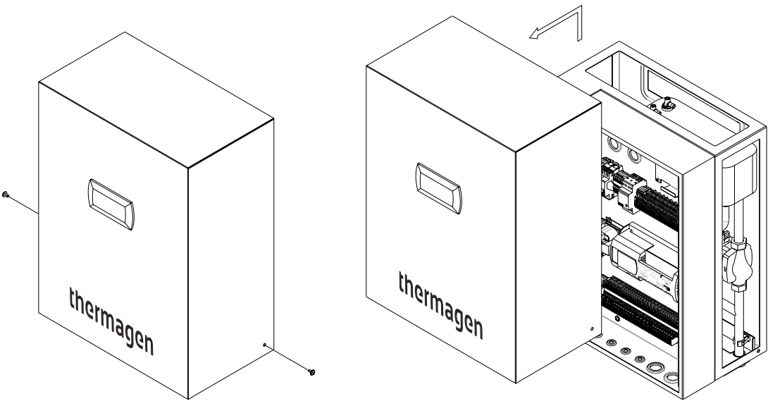
Ilustracja 3.3. Demontaż osłon modułu wewnętrznego Intra HEX.
