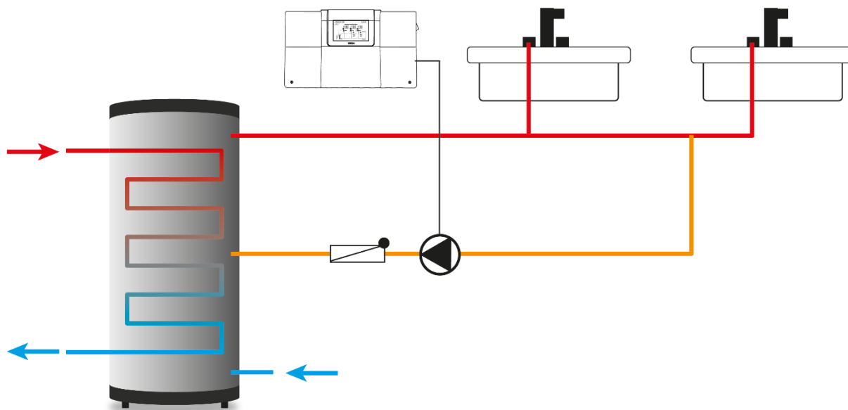
Przykładowe połączenie i sterowanie pracą pompy cyrkulacyjnej
