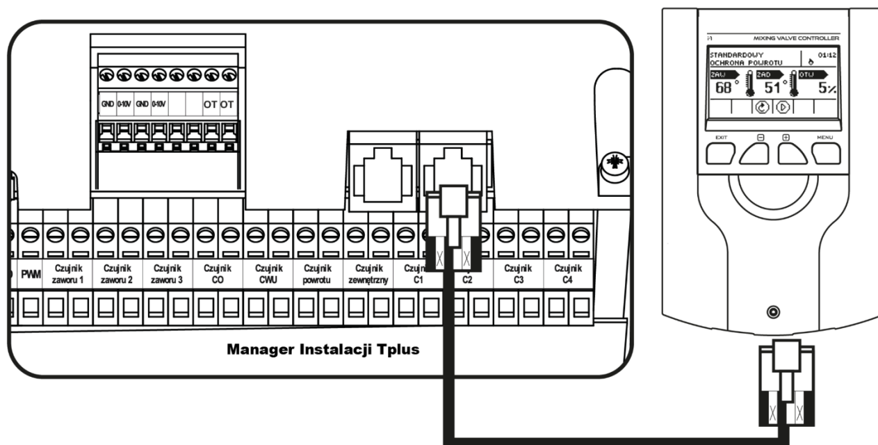
Przykładowe podłączenie zaworu dodatkowego ze sterownikiem głównym
