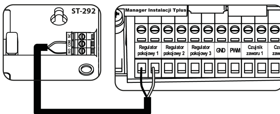
Przykładowe podłączenie regulatora dwustanowego
